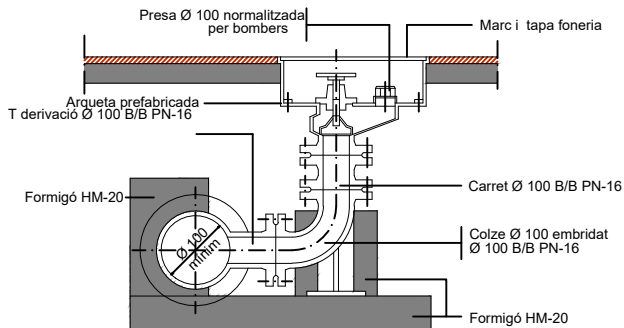
HIDRANT SOTERRAT
