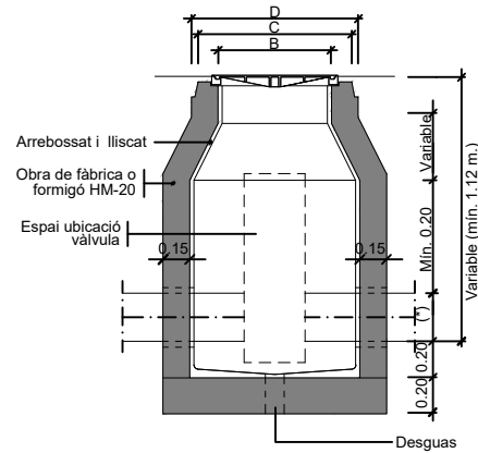
ARQUETA TIPUS II
