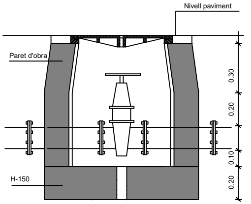
SECCIÓ
