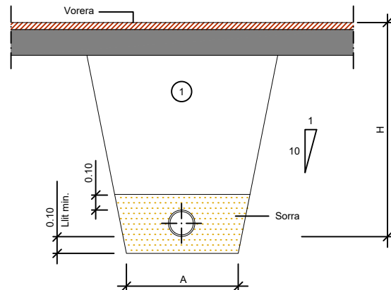
RASA PER A CONDUCCIÓ SOTA VORERA
