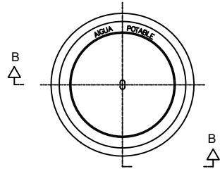
PLANTA TAPA
