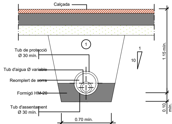
RASA PER A CONDUCCIÓ SOTA VIAL
