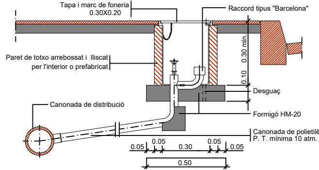
BOCA DE REG Ø 45MM.
