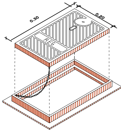
MARC I TAPA, DE FONÈRIA PER A BOCA DE REG
