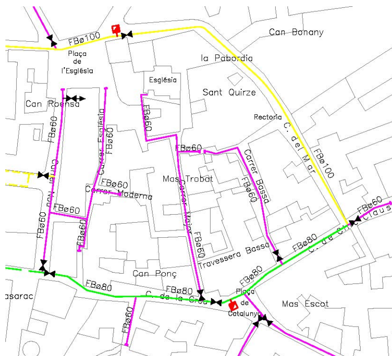
Estat actual xarxa pública d'aigua potable en el nucli de Viladamat
