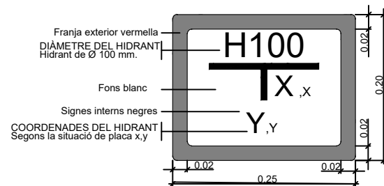
PLACA VERTICAL DE SENYALITZACIÓ D'HIDRANT SOTERRAT
